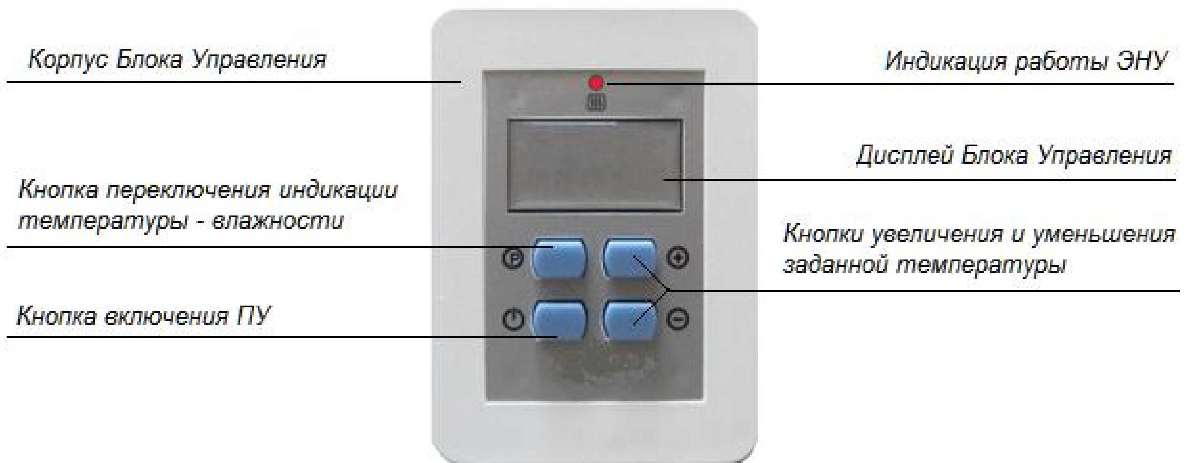
Рис. 2.5.2. Блок управления ПУ-04М
