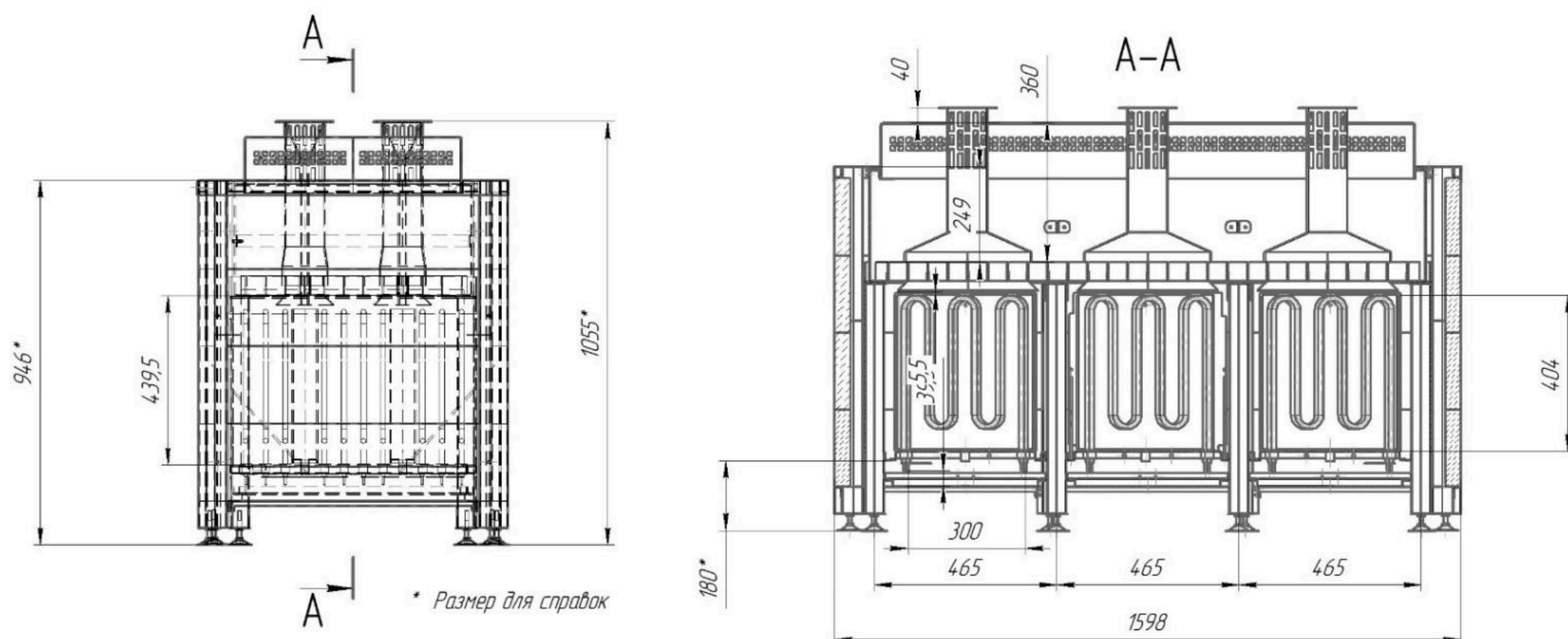
Рис. 1.2.3. Внешний вид Электропечи при трехсекционном исполнении (в разрезе)
