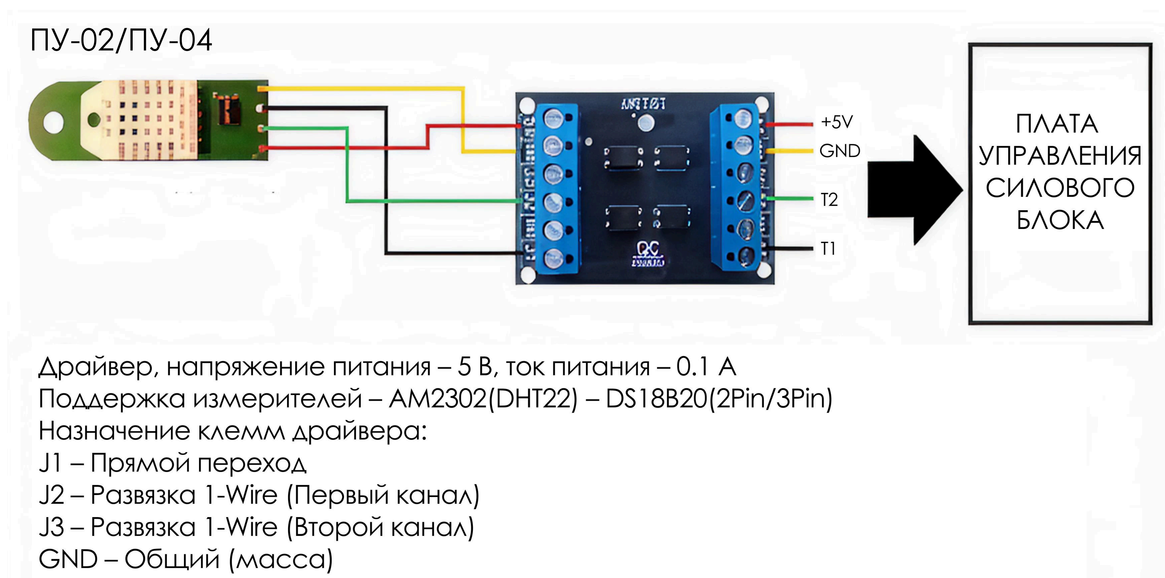
Рис. 1.4.1. Драйвер датчика температуры и влажности
