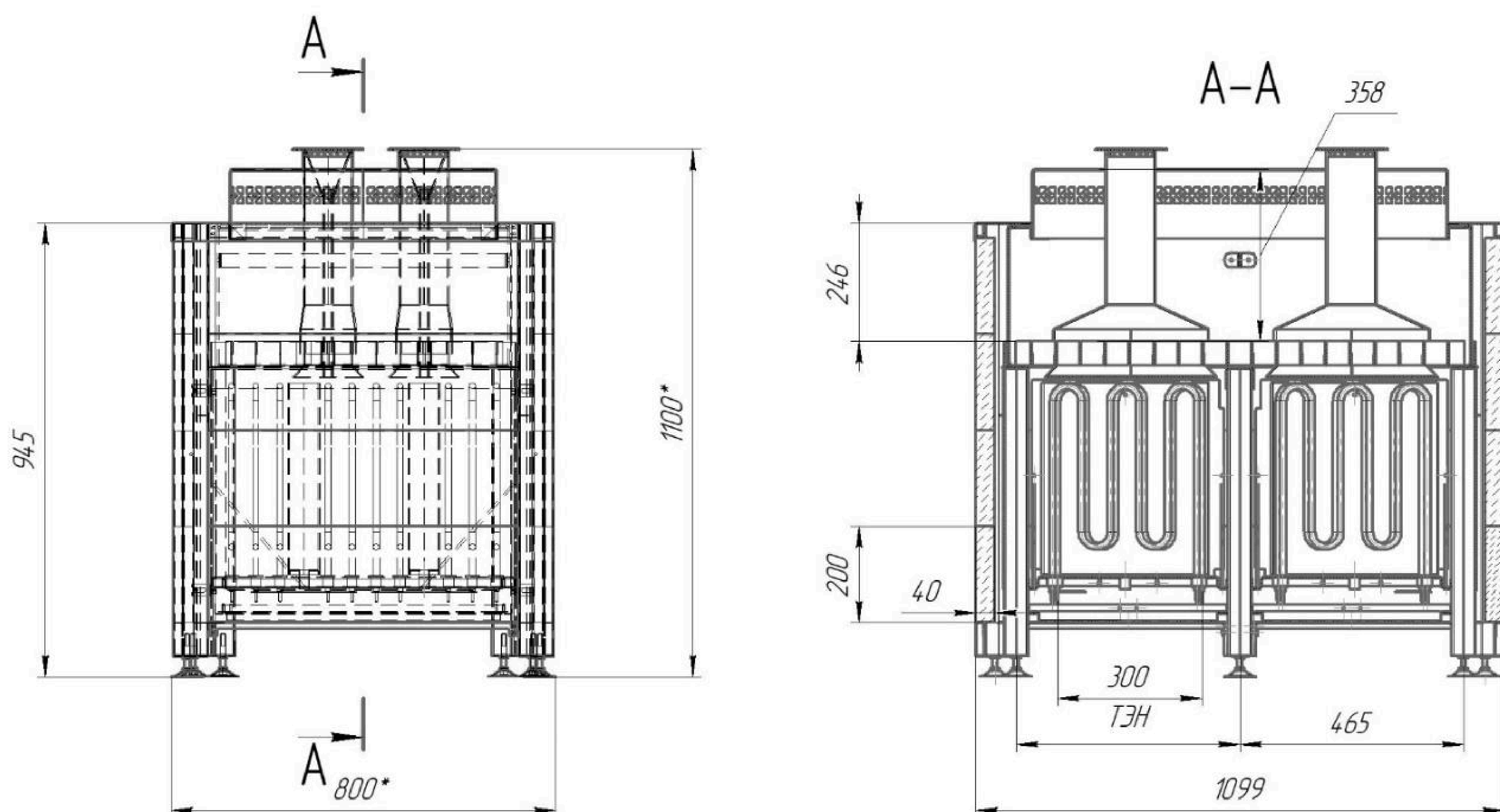
Рис. 1.2.2. Внешний вид Электropечи при двухсекционном исполнении (в разрезе)
