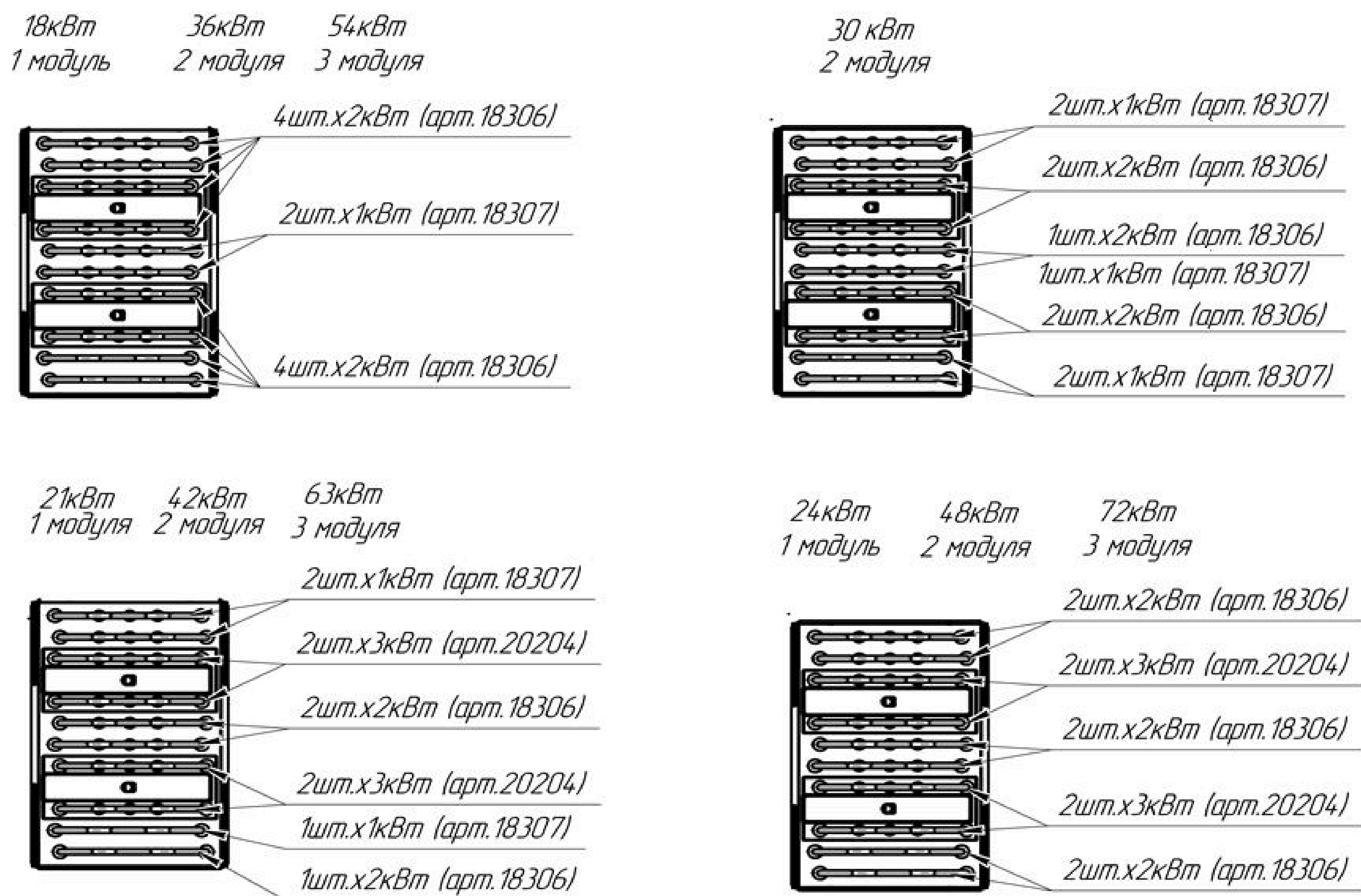
Рис. 1.3.1. Компоновка, мощность и количество ТЭНов в модулях ЭН «Премьера-Профи»
