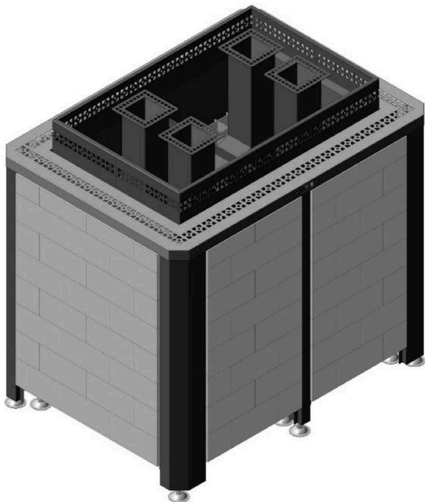
Рис. 2. Сборка ЭНУ Премьера Профи Гималайская соль
