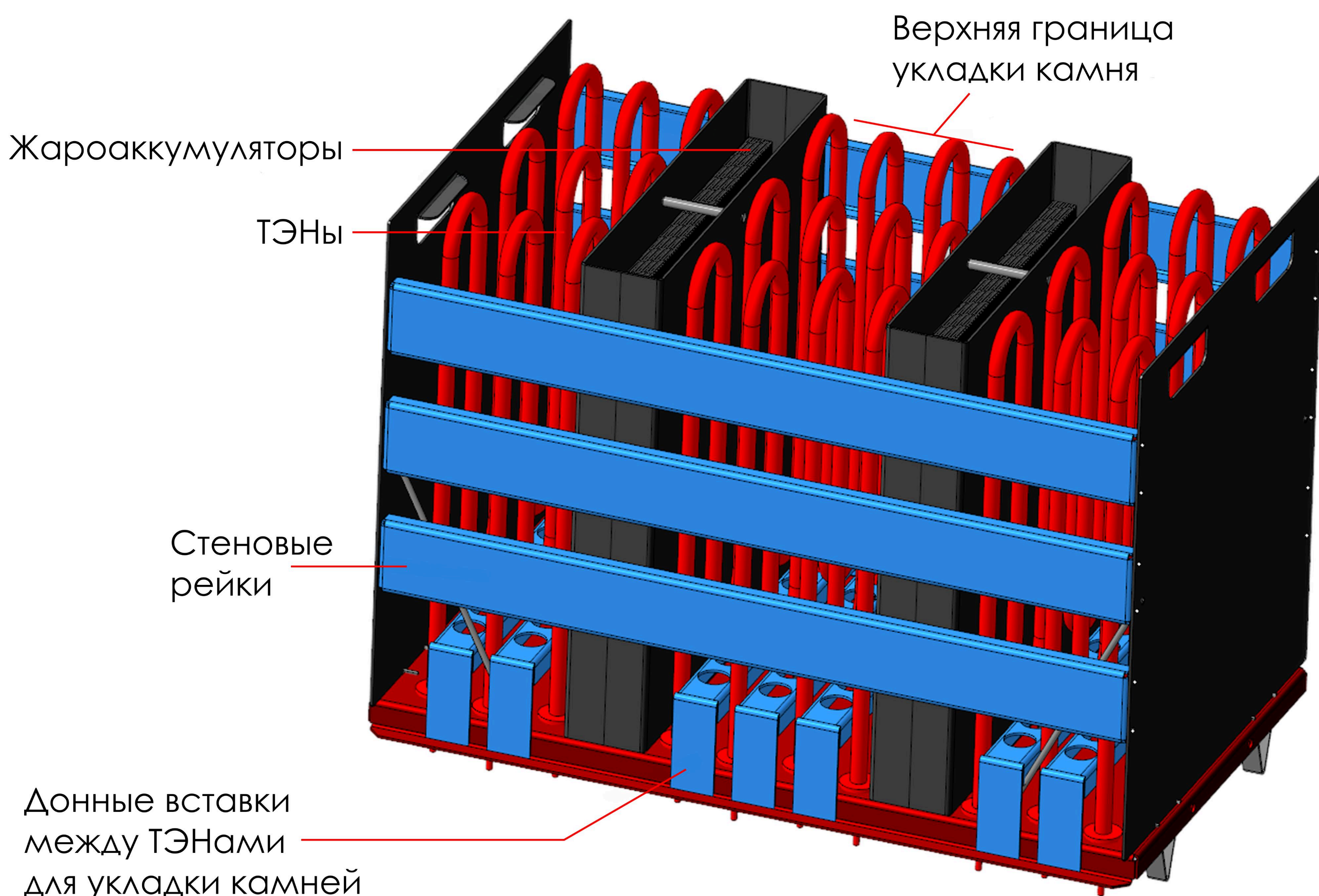
Рис. 1.4. Блок ТЭНов Электрической печи Премьера Профи
