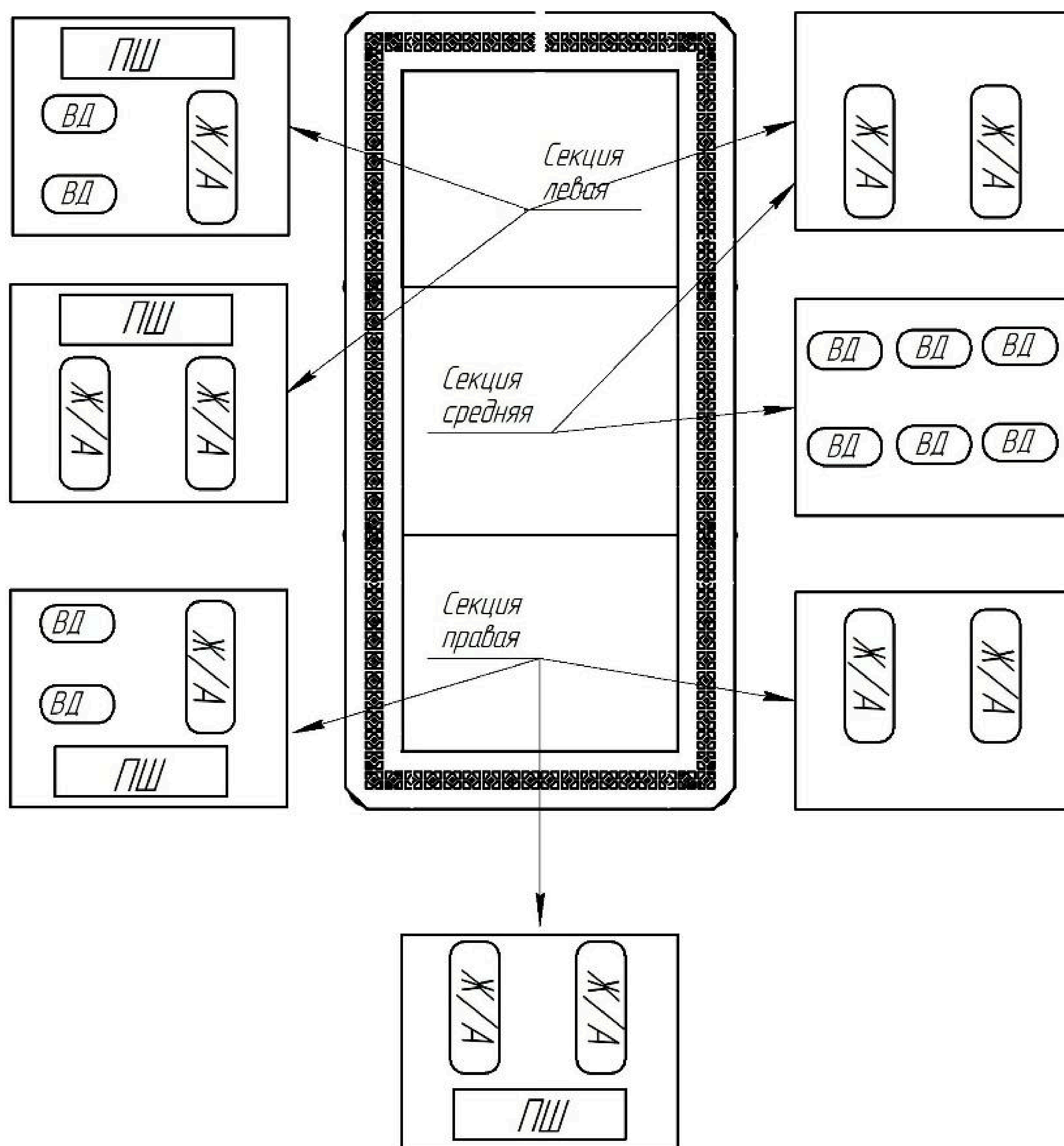
Схема 3. Премьера Профи в 3-х секционном исполнении
