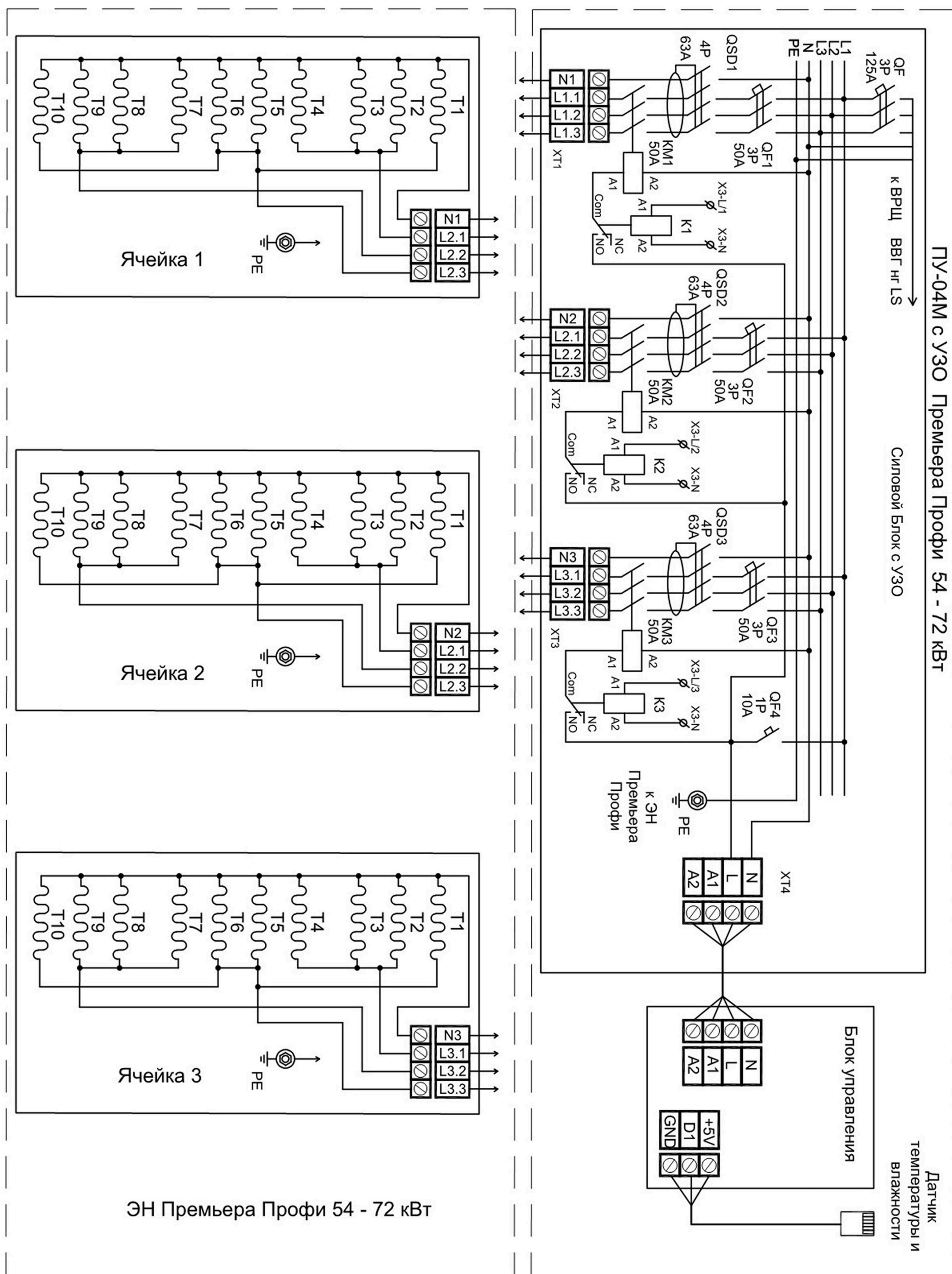
Рис. 1.3.9. Подключение ЭН и ПУ-04М к электрической сети при односекционном исполнении 54-72 кВт
