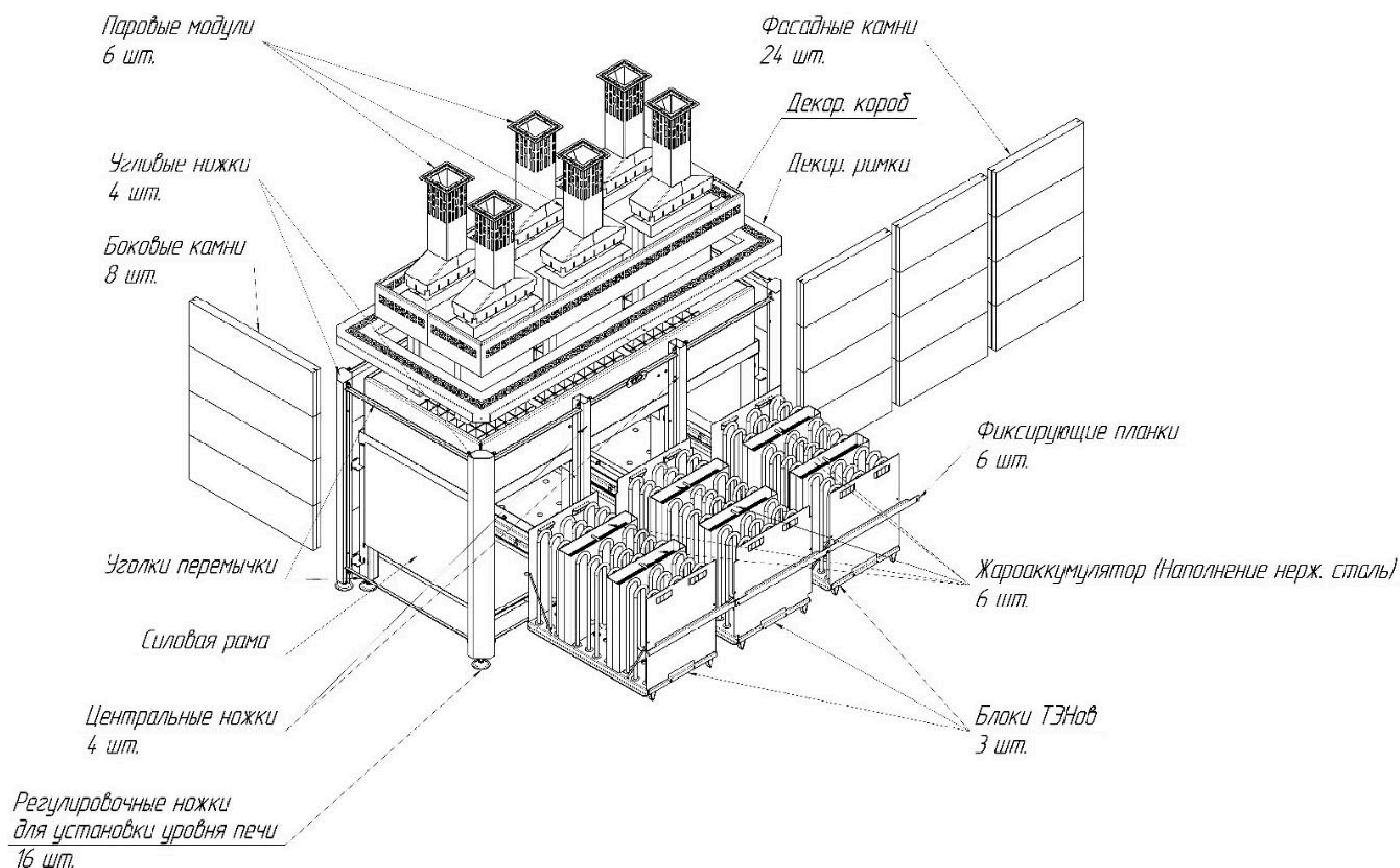
Рис. 1. Сборка ЭНУ Премьера Профи в каменной облицовке
