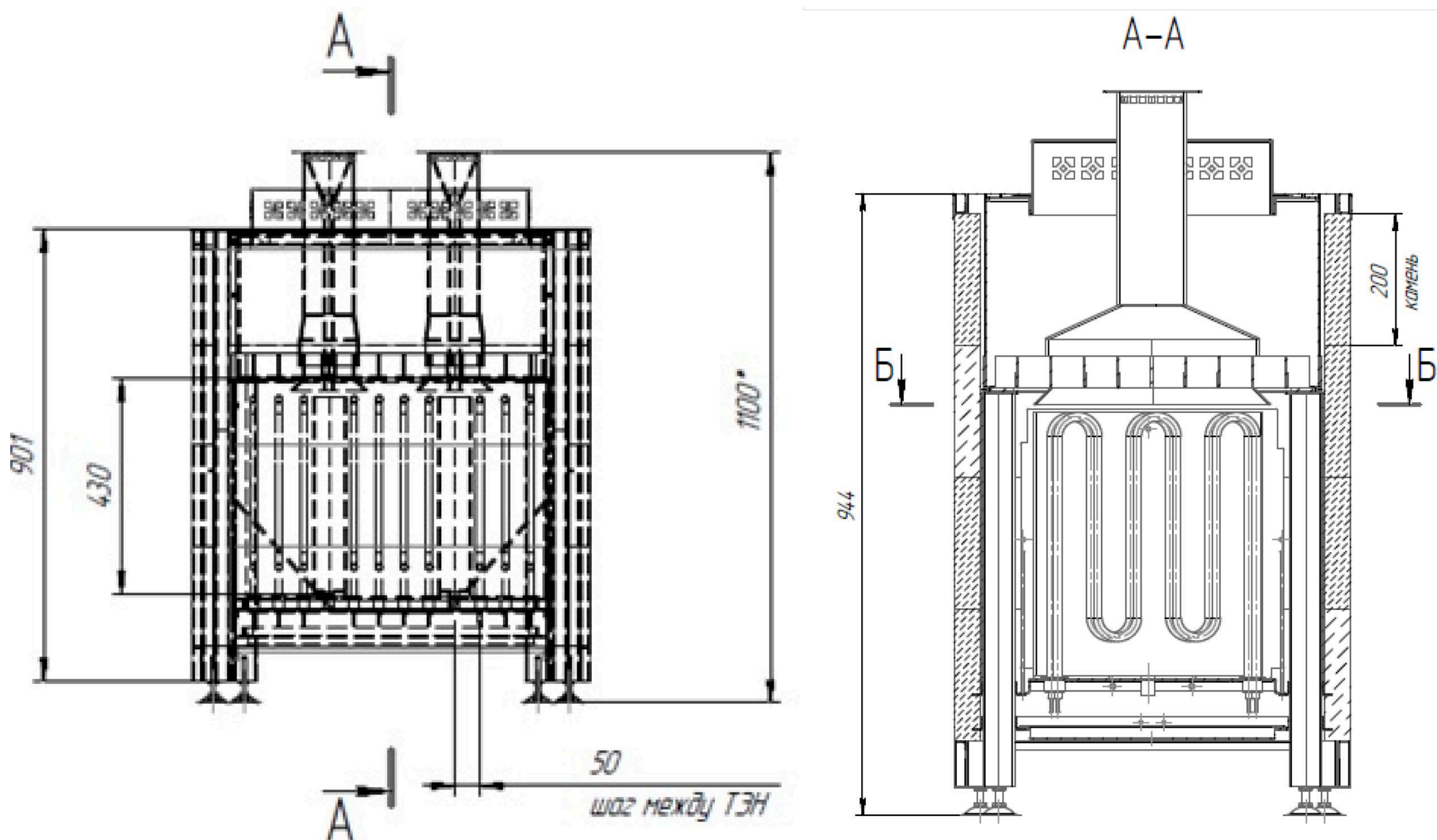
Рис. 1.2.1. Внешний вид Электropечи при односекционном исполнении (в разрезе)
