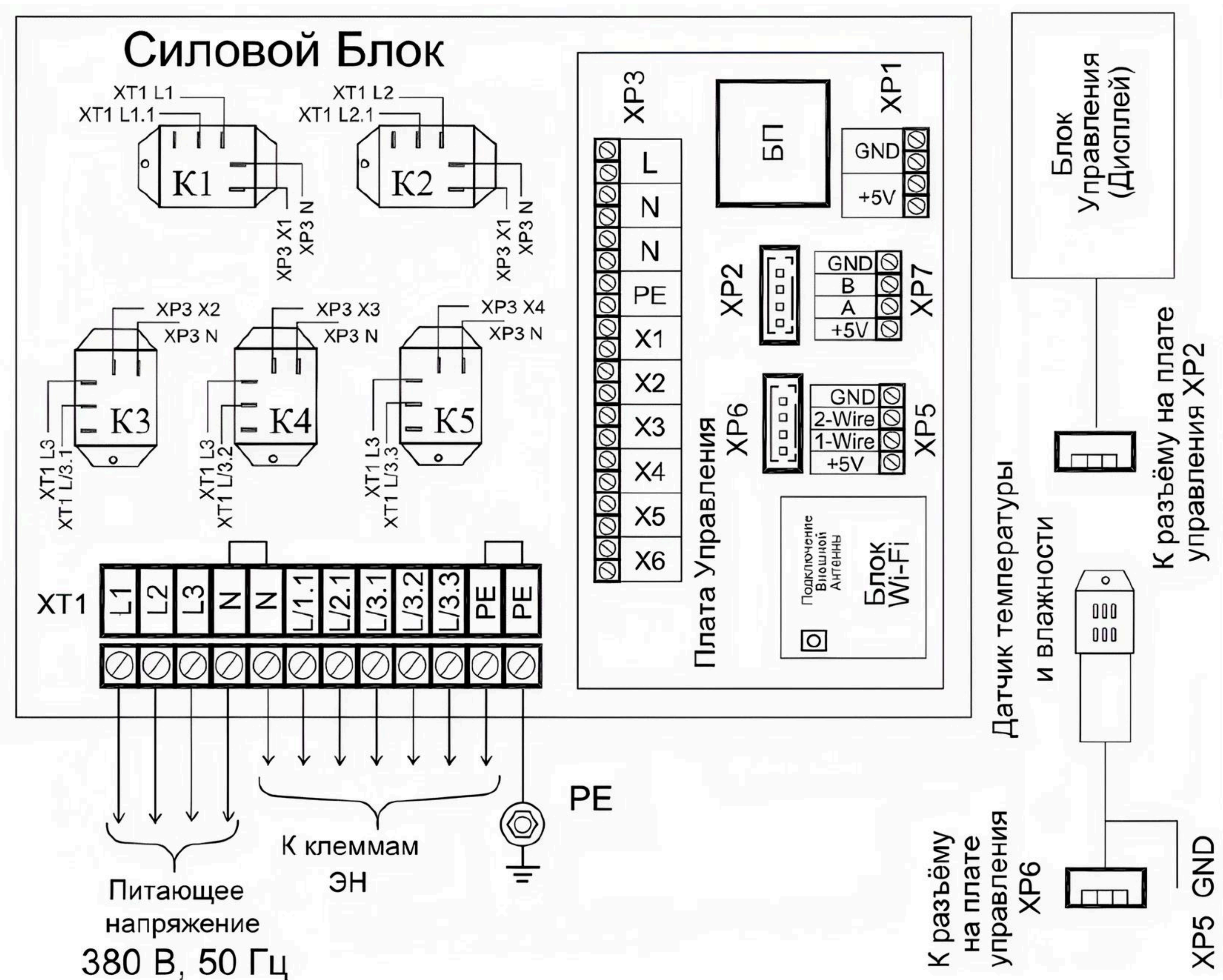
Рис. 8. Схема электрических подключений ПУ-09 МП ВВД Про 4,25-6,25/380
