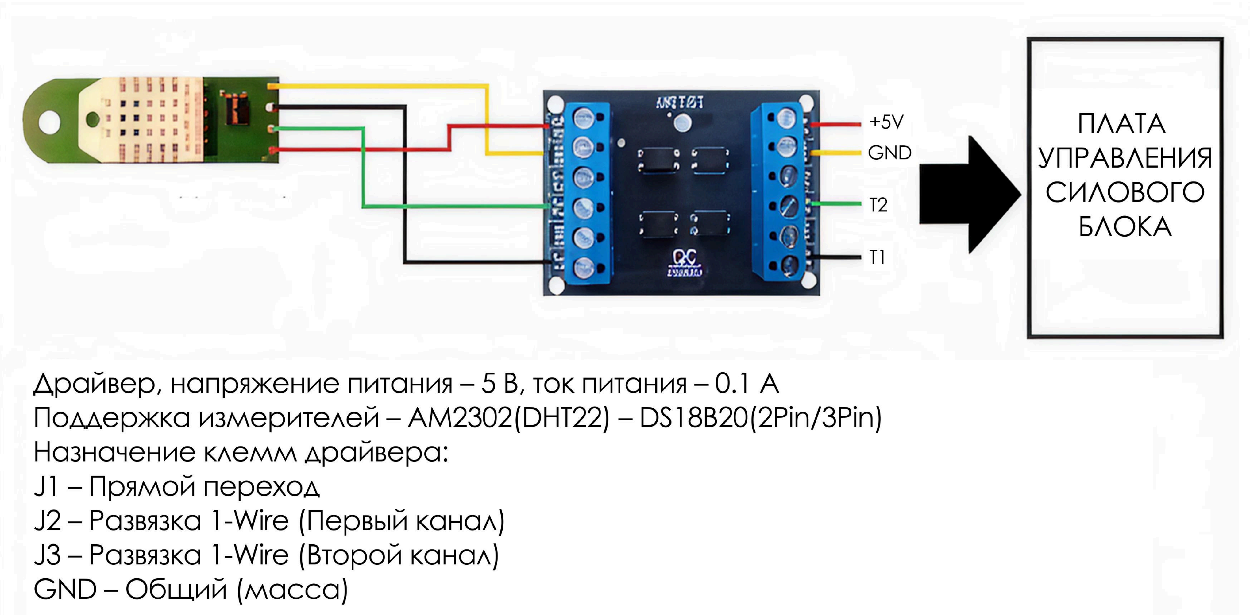
Рис. 3. Драйвер (усилитель сигнала) датчика температуры и влажности
