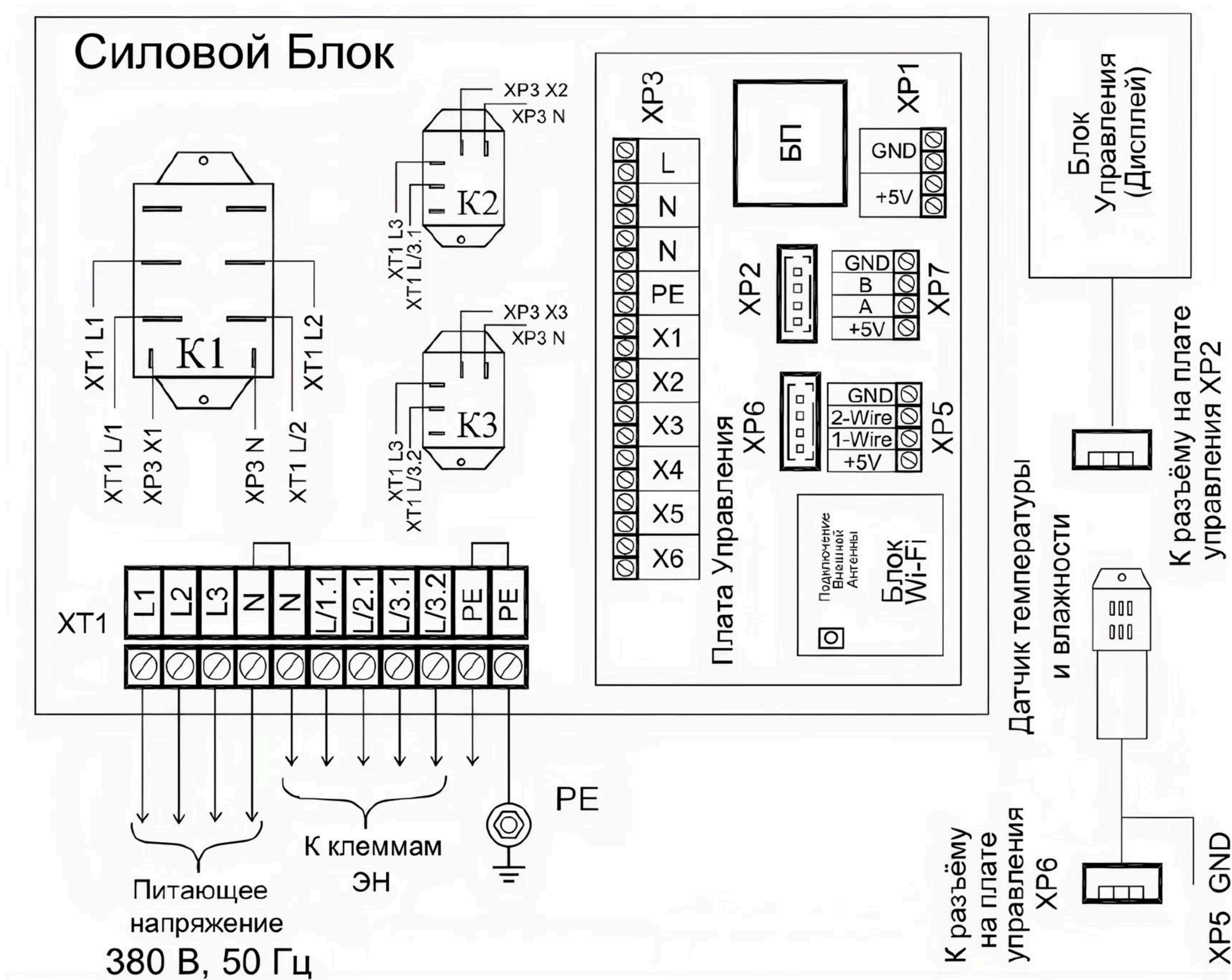
Рис. 9. Схема электрических подключений ПУ-09 ВВД Про 10-24/380
