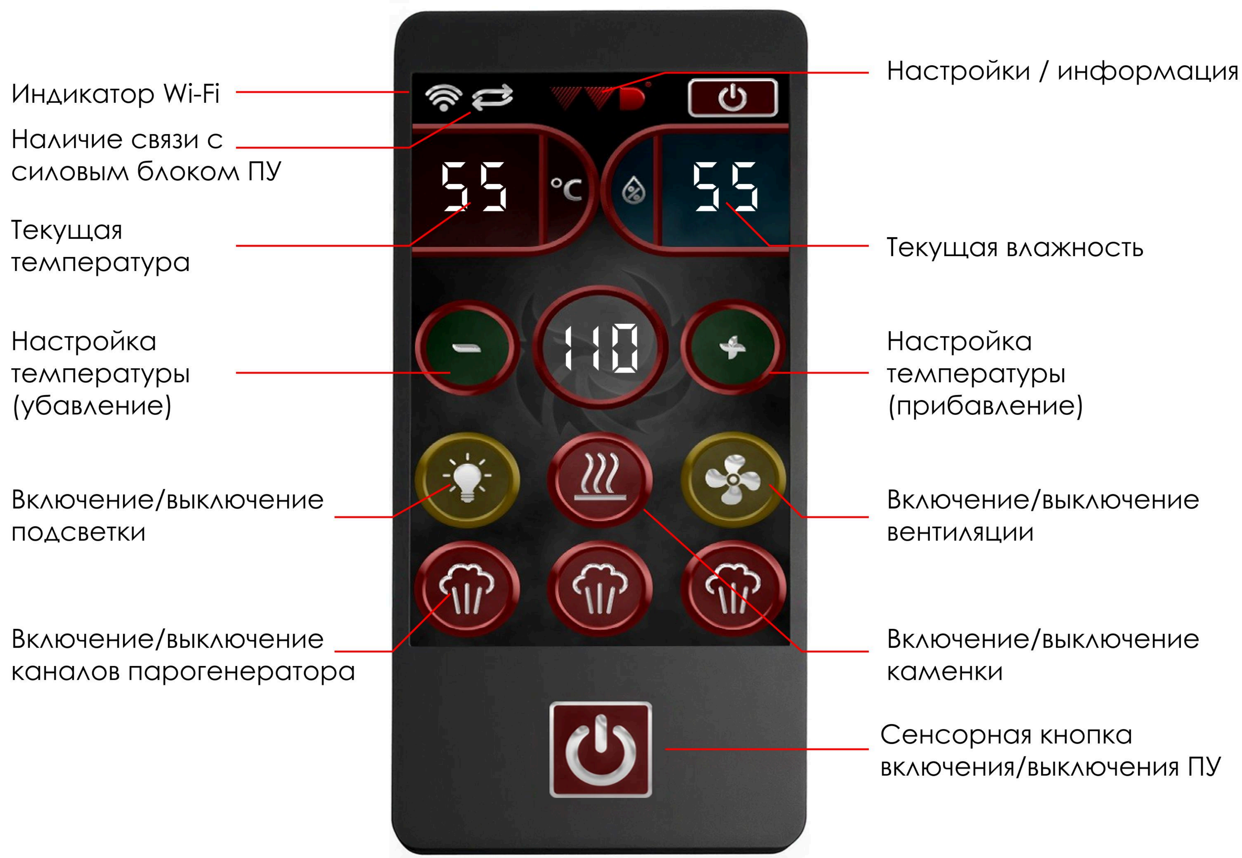
Рис. 10. Блок управления ПУ-08.1 и ПУ-09
